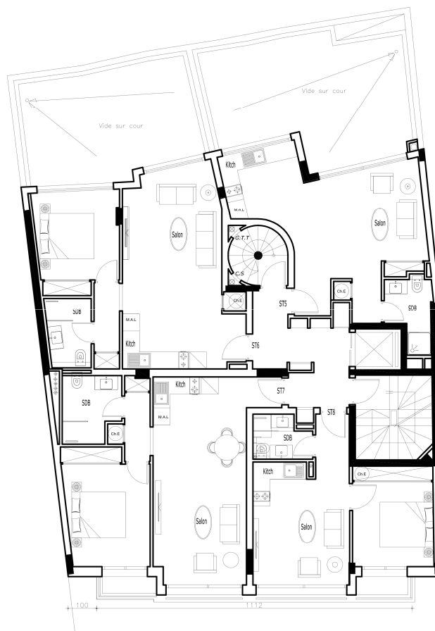
2ème ETAGE
