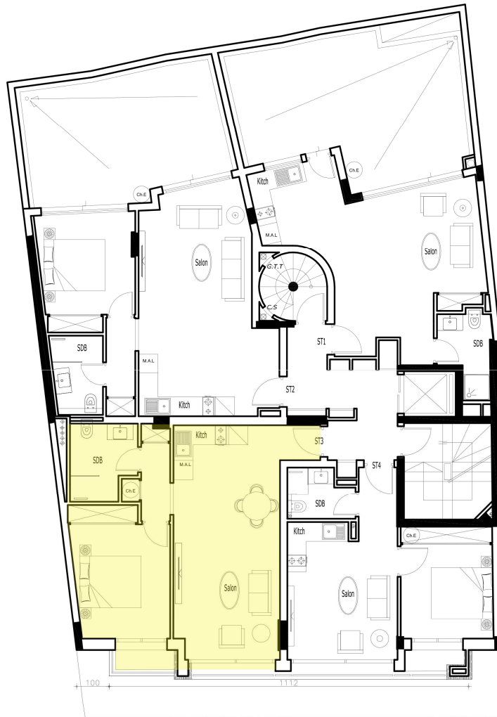
1er ETAGE
