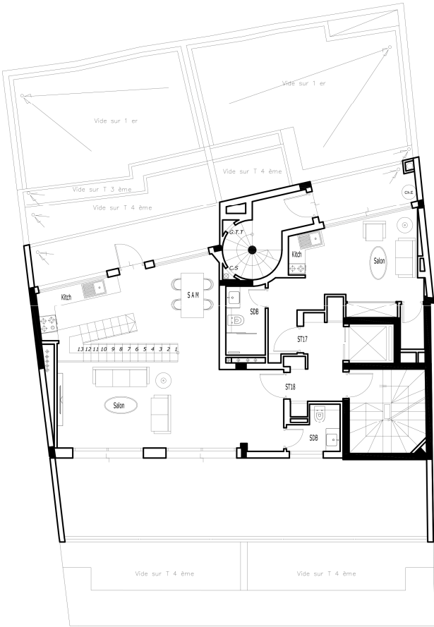
5ème ETAGE
